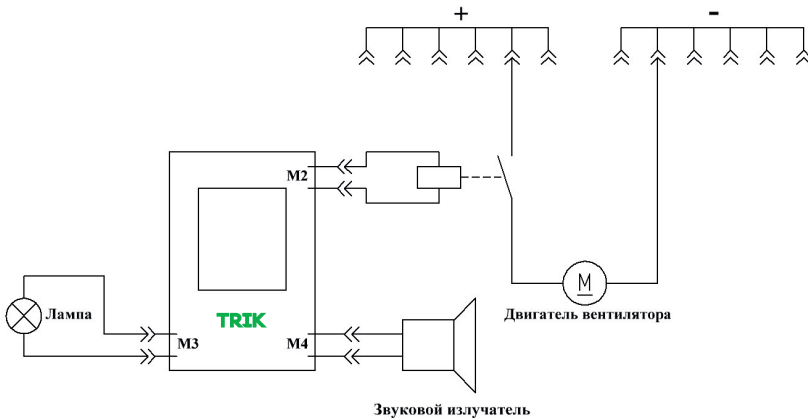
Подключение элементов стенда
