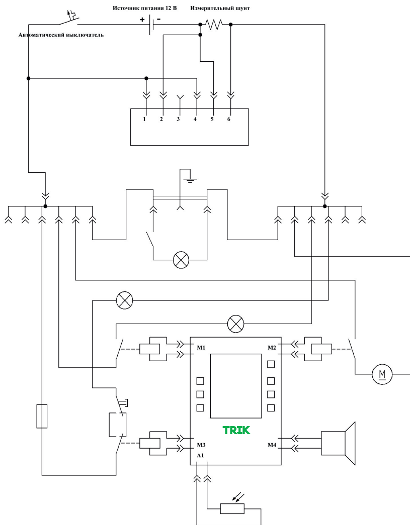
Общая принципиальная электрическая схема:
