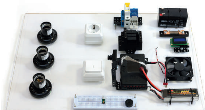
Собранный стенд «Электротехника»
