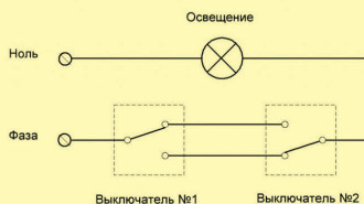
Схема проходного выключателя
