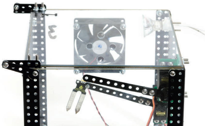
Крепление щупа датчика влажности почвы
