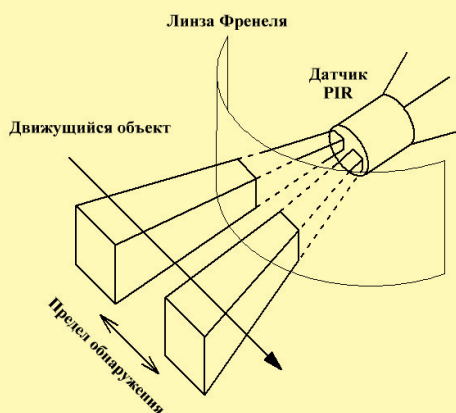
Принцип работы PIR датчика
