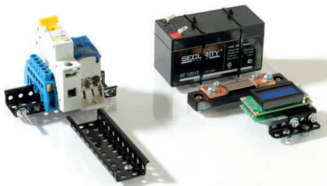
Крепление распределительных шин, автоматического выключателя и заземления
