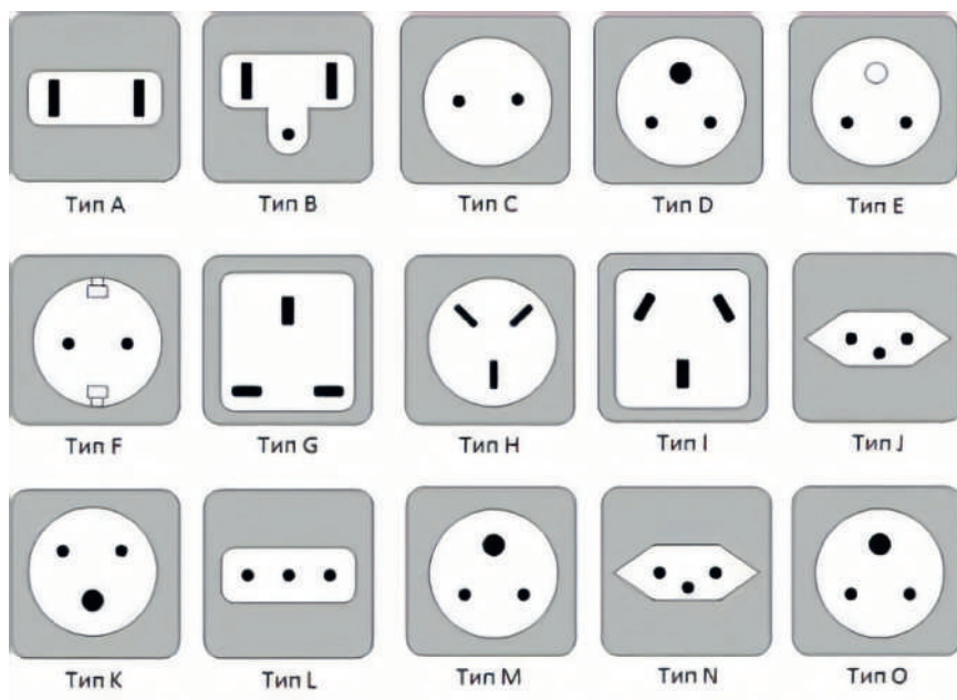
Типы розеток
