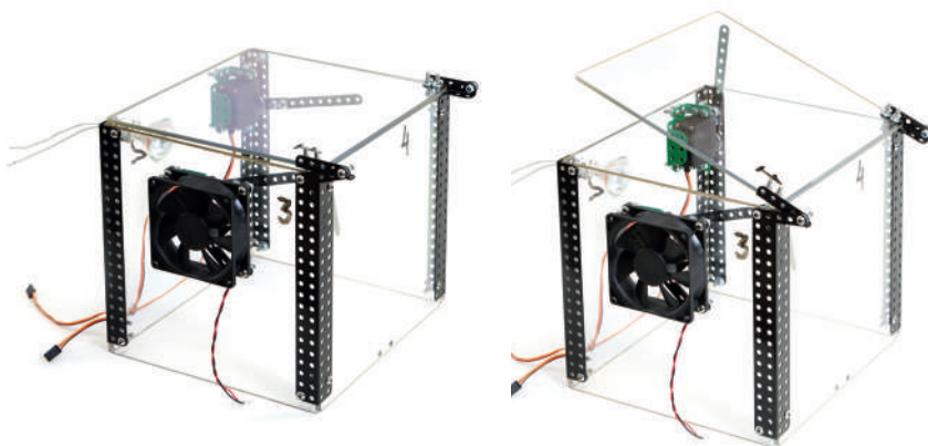
Различные положения крышки теплицы
