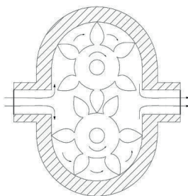
Шестеренчатый насос
