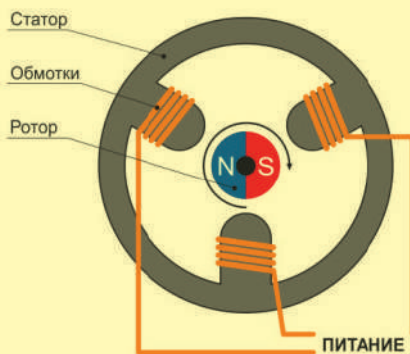
Принцип работы бесколлекторного мотора
