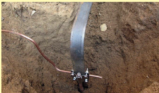
Заземление
