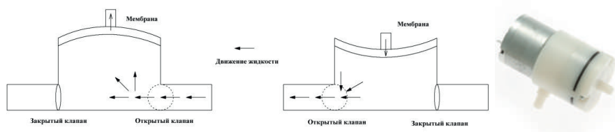
Мембранный насос
