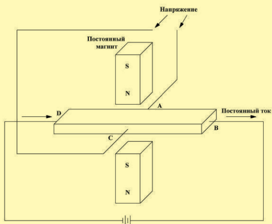
Схема, собранная Холлом
