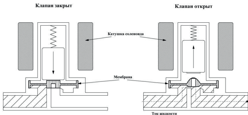
Схема работы электромагнитного клапана
