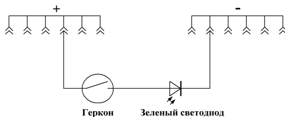
Схема «Сигнализация о проникновении»
