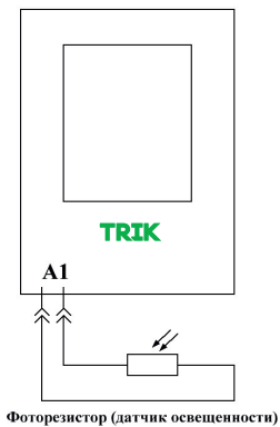
Подключение датчика освещенности
