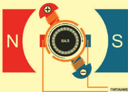
Принцип работы коллекторного двигателя
