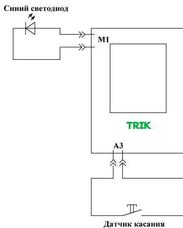
Схема «Двери закрыты»
