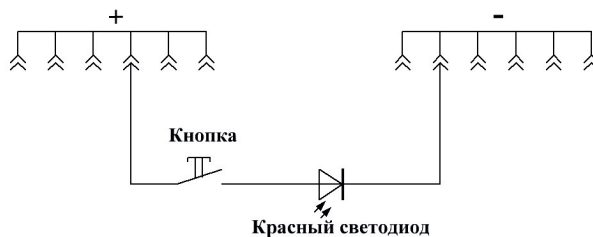
Схема «Сигнал тревоги»
