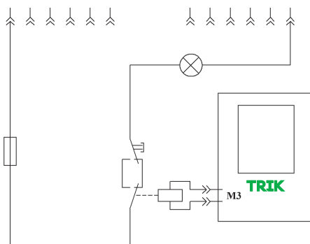
Проходной выключатель
