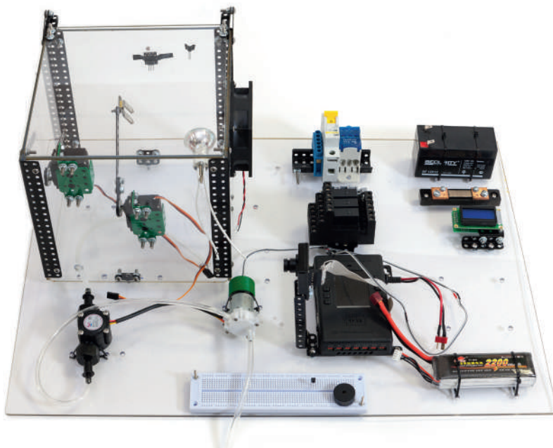
Собранный стенд «Грядка»
