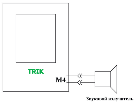
Подключение пьезоизлучателя
