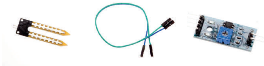
Щуп, соединительный провод и датчик влажности почвы
