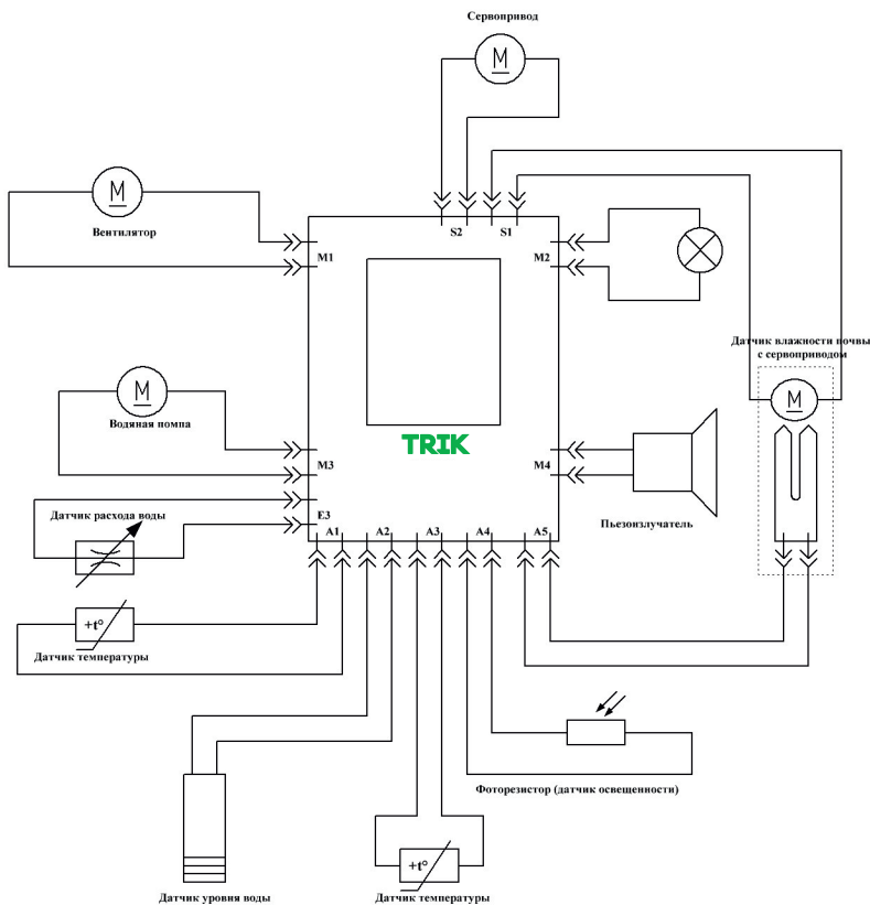
Схема подключения элементов теплицы
