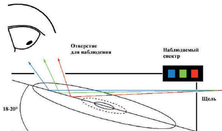
Использование CD диска в качестве дифракционной решетки
