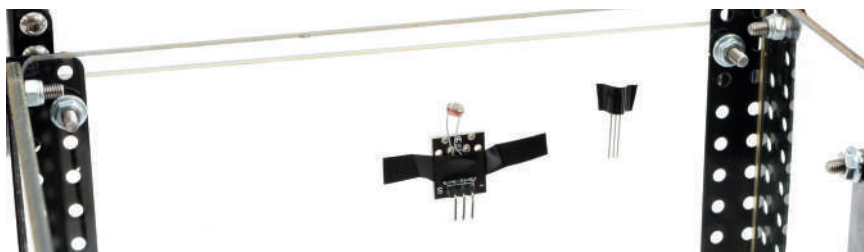
Крепление датчиков освещенности и температуры
