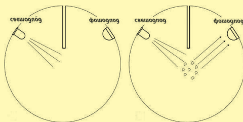
Принцип работы точечного дымового извещателя
