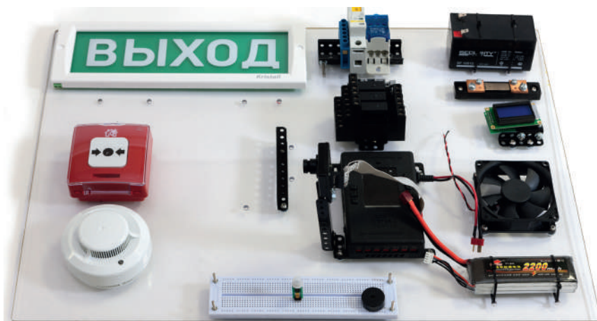
Собранный стенд «Пожарная и охранная сигнализация»
