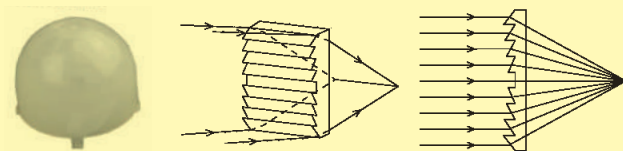
Линза Френеля
