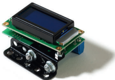
Дополнительная конструкция для крепления амперметра-вольтметра
